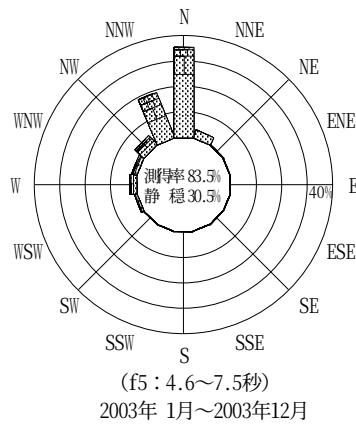
図-12.6 新潟沖 波高・波向別出現頻度図 (f2, f3, f4, f5, 全周期帯)
