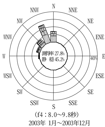
図-12.11 金沢 波高・波向別出現頻度図 (f2, f3, f4, f5, 全周期帯)
