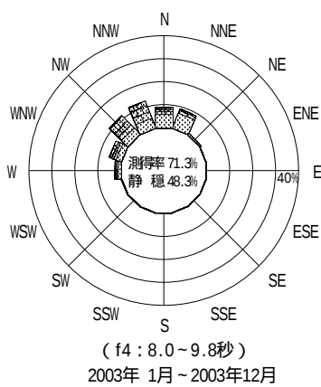
図 - 12.10 輪島 波高・波向別出現頻度図 ( f2 , f3 , f4 , f5 , 全周期帯 )
