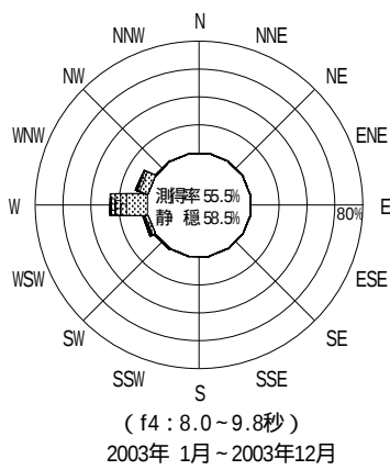
図 - 12.4 秋田 波高・波向別出現頻度図 ( f2 , f3 , f4 , f5 , 全周期帯 )
