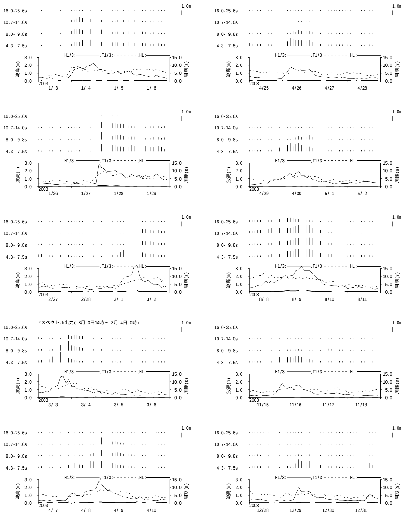
図 - 11.36 アシカ島 周期帯別波浪特性の経時変化(高波期間中)
