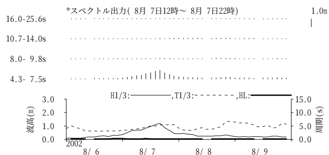
図-11.55 石垣 周期帯別波浪特性の経時変化(高波期間中)
