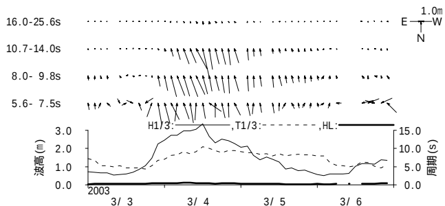
図 - 11.21 那覇 周期帯別波浪特性の経時変化(高波期間中)
