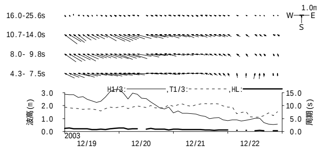
図 - 11.23 十勝 周期帯別波浪特性の経時変化(高波期間中)
