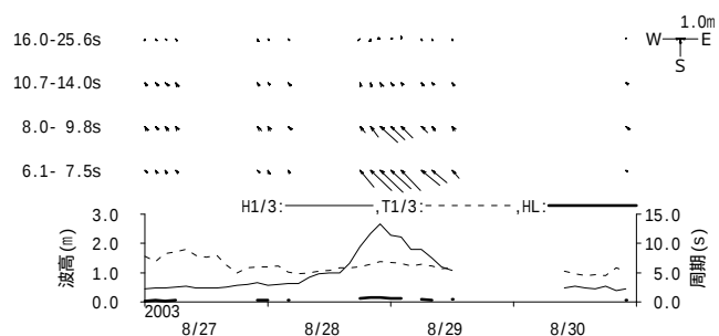
図 - 11.24 苫小牧 周期帯別波浪特性の経時変化(高波期間中)
