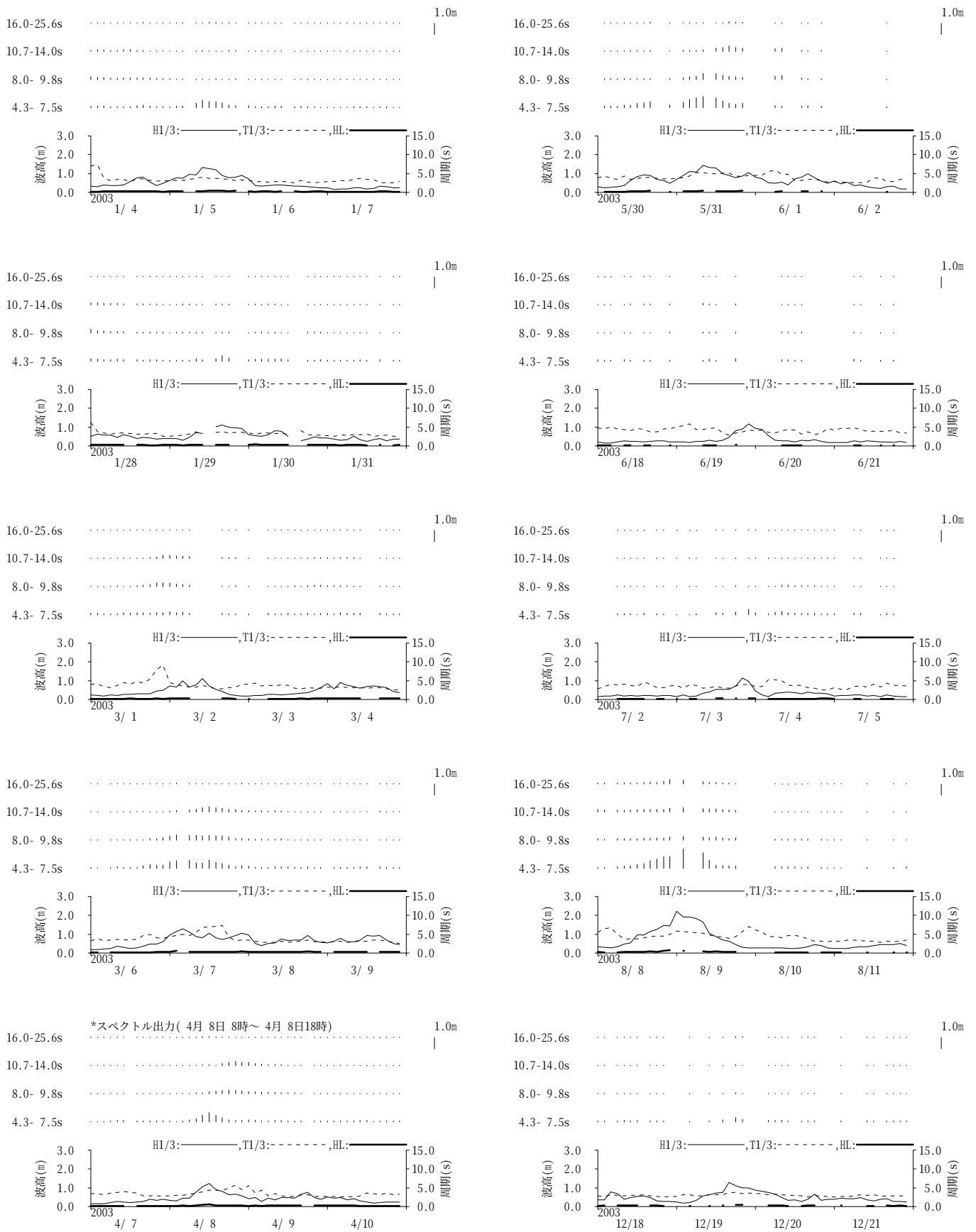
図-11.41 伊勢湾 周期帯別波浪特性の経時変化(高波期間中)
