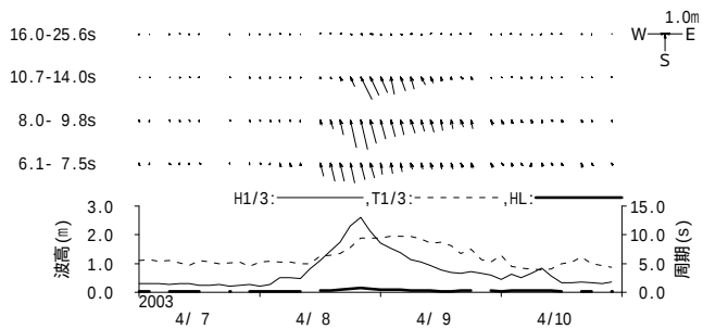
図 - 11.39 清水 周期帯別波浪特性の経時変化(高波期間中)
