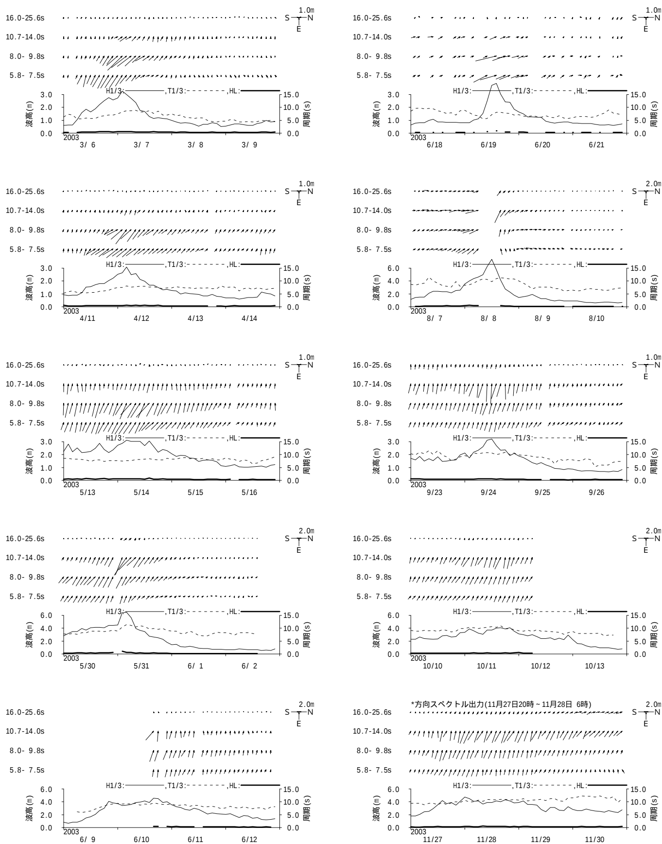
図 - 11.49 細島 周期帯別波浪特性の経時変化(高波期間中)
