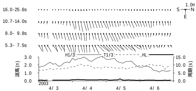
図 - 11.50 宮崎 周期帯別波浪特性の経時変化(高波期間中)
