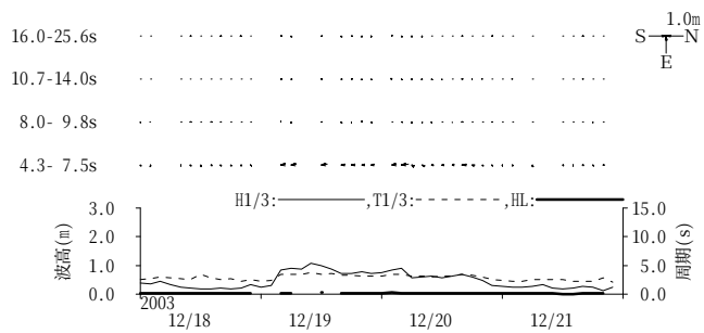
図-11.48 荻田 周期帯別波浪特性の経時変化(高波期間中)
