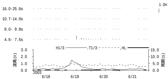
図 - 11.52 鹿児島 周期帯別波浪特性の経時変化(高波期間中)
