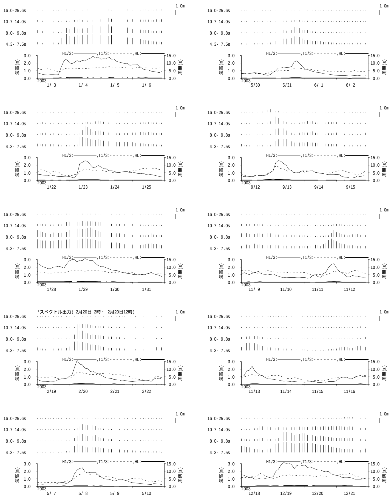
図 - 11.17 藍島 周期帯別波浪特性の経時変化(高波期間中)
