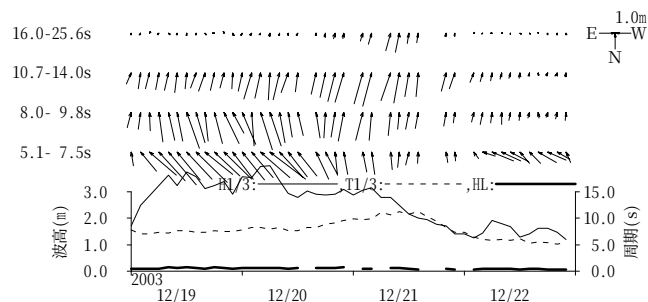
図-11.18 玄界灘 周期帯別波浪特性の経時変化(高波期間中)
