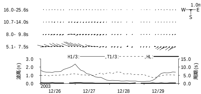
図 - 11.19 伊王島 周期帯別波浪特性の経時変化(高波期間中)
