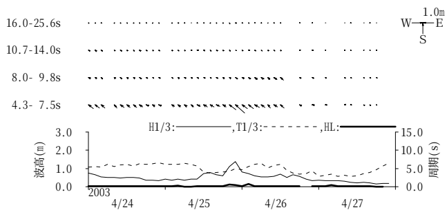
図-11.44 小松島 周期帯別波浪特性の経時変化(高波期間中)
