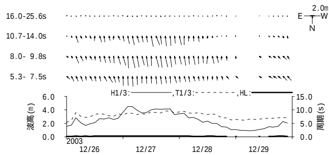
図 - 11.12 柴山 周期帯別波浪特性の経時変化(高波期間中)
