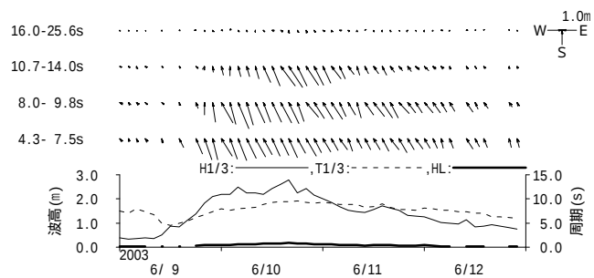
図 - 11.46 高知 周期帯別波浪特性の経時変化(高波期間中)
