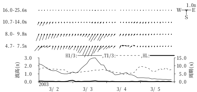
図-11.45 室津 周期帯別波浪特性の経時変化(高波期間中)
