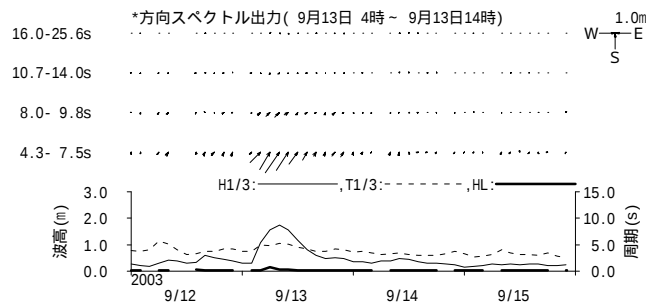
図 - 11.43 神戸 周期帯別波浪特性の経時変化(高波期間中)
