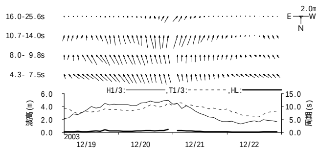
図 - 11.14 鳥取 周期帯別波浪特性の経時変化(高波期間中)
