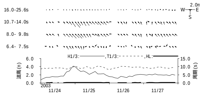
図 - 11.42 潮岬 周期帯別波浪特性の経時変化(高波期間中)
