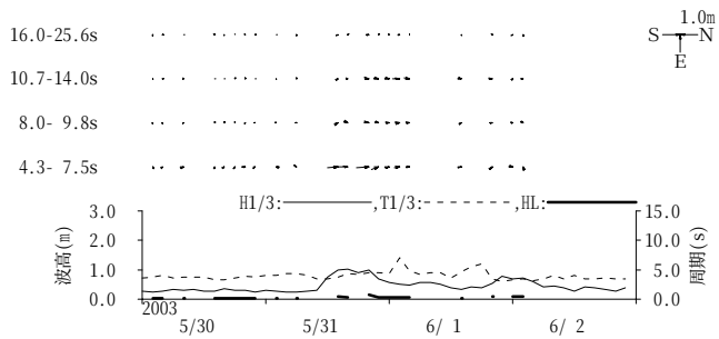
図-11.35 第二海堡 周期帯別波浪特性の経時変化(高波期間中)
