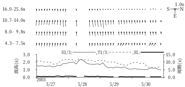
図-11.31 相馬 周期帯別波浪特性の経時変化(高波期間中)
