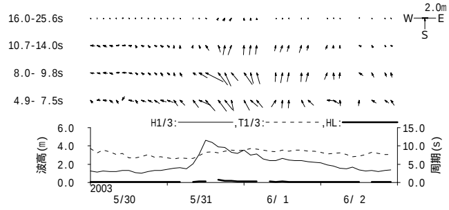
図 - 11.37 波浮 周期帯別波浪特性の経時変化(高波期間中)
