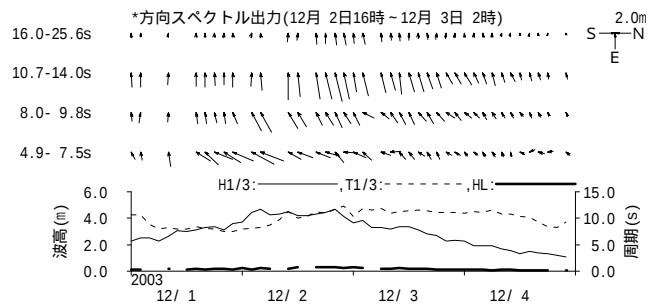
図 - 11.33 常陸那珂 周期帯別波浪特性の経時変化(高波期間中)
