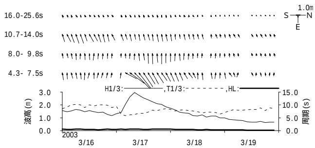
図 - 11.34 鹿島 周期帯別波浪特性の経時変化(高波期間中)
