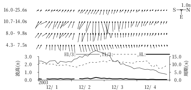
図-11.32 小名浜 周期帯別波浪特性の経時変化(高波期間中)
