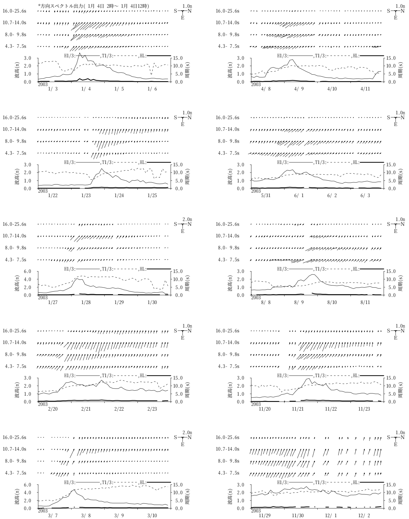
図-11.30 仙台新港 周期帯別波浪特性の経時変化(高波期間中)
