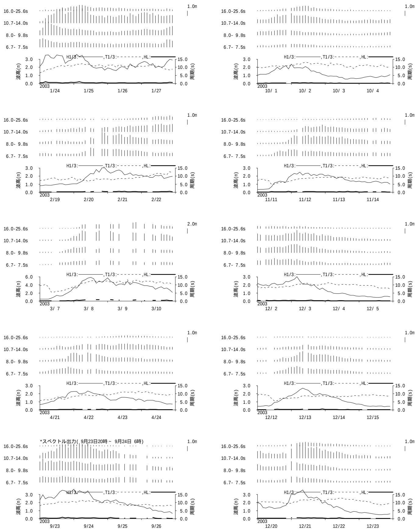
図 - 11.28 釜石 周期帯別波浪特性の経時変化(高波期間中)
