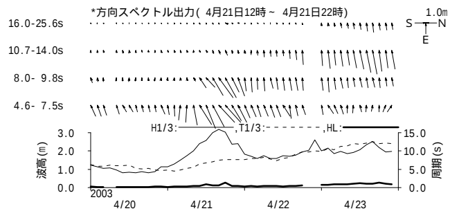
図 - 11.26 八戸 周期帯別波浪特性の経時変化(高波期間中)
