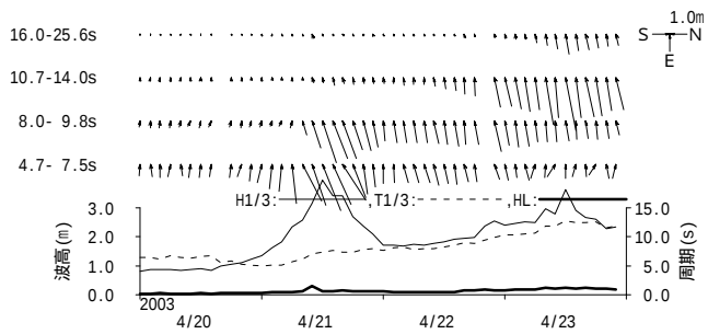
図 - 11.25 むつ小川原 周期帯別波浪特性の経時変化(高波期間中)
