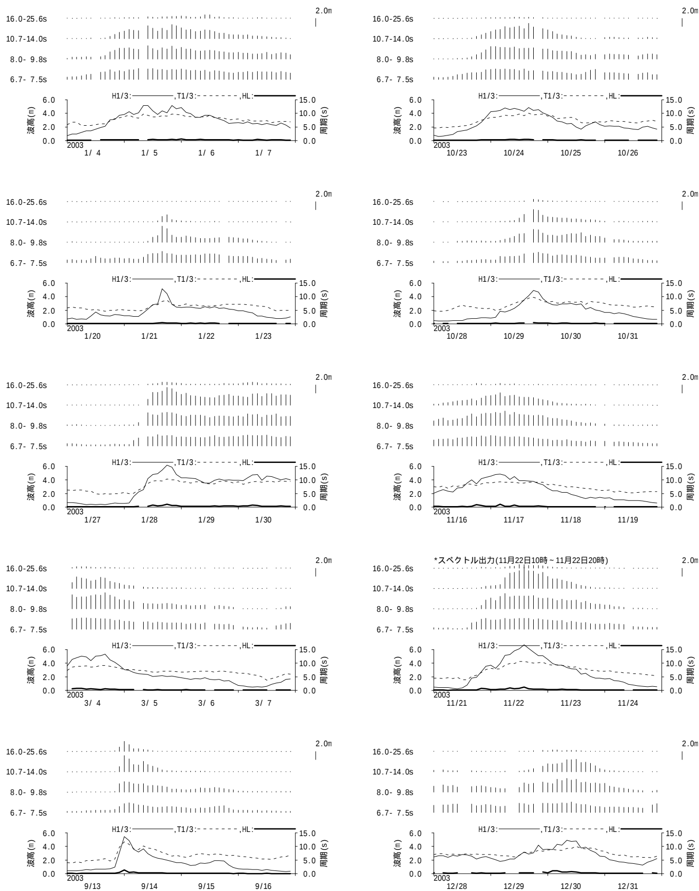
図 - 11.3 深浦 周期帯別波浪特性の経時変化(高波期間中)
