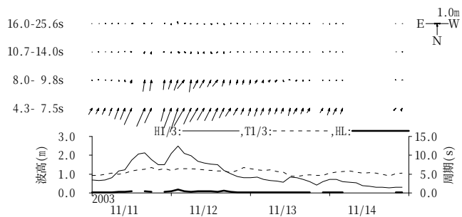
図-11.8 富山 周期帯別波浪特性の経時変化(高波期間中)
