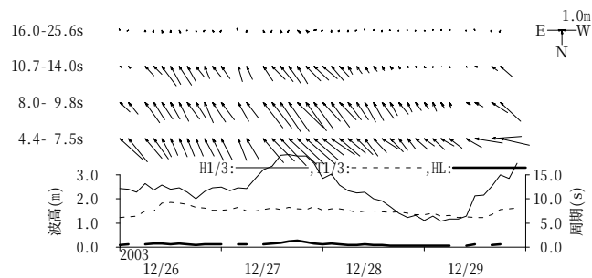
図-11.7 直江津 周期帯別波浪特性の経時変化(高波期間中)
