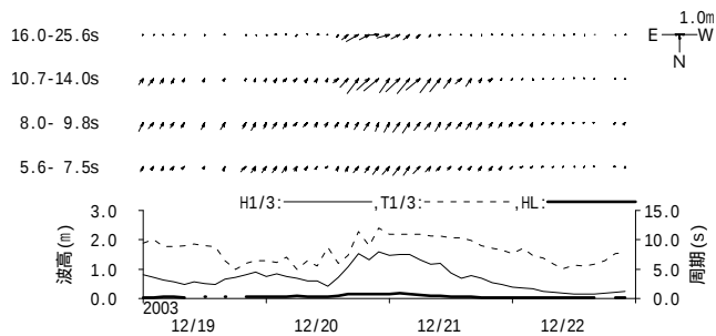
図 - 11.9 伏木富山 周期帯別波浪特性の経時変化(高波期間中)
