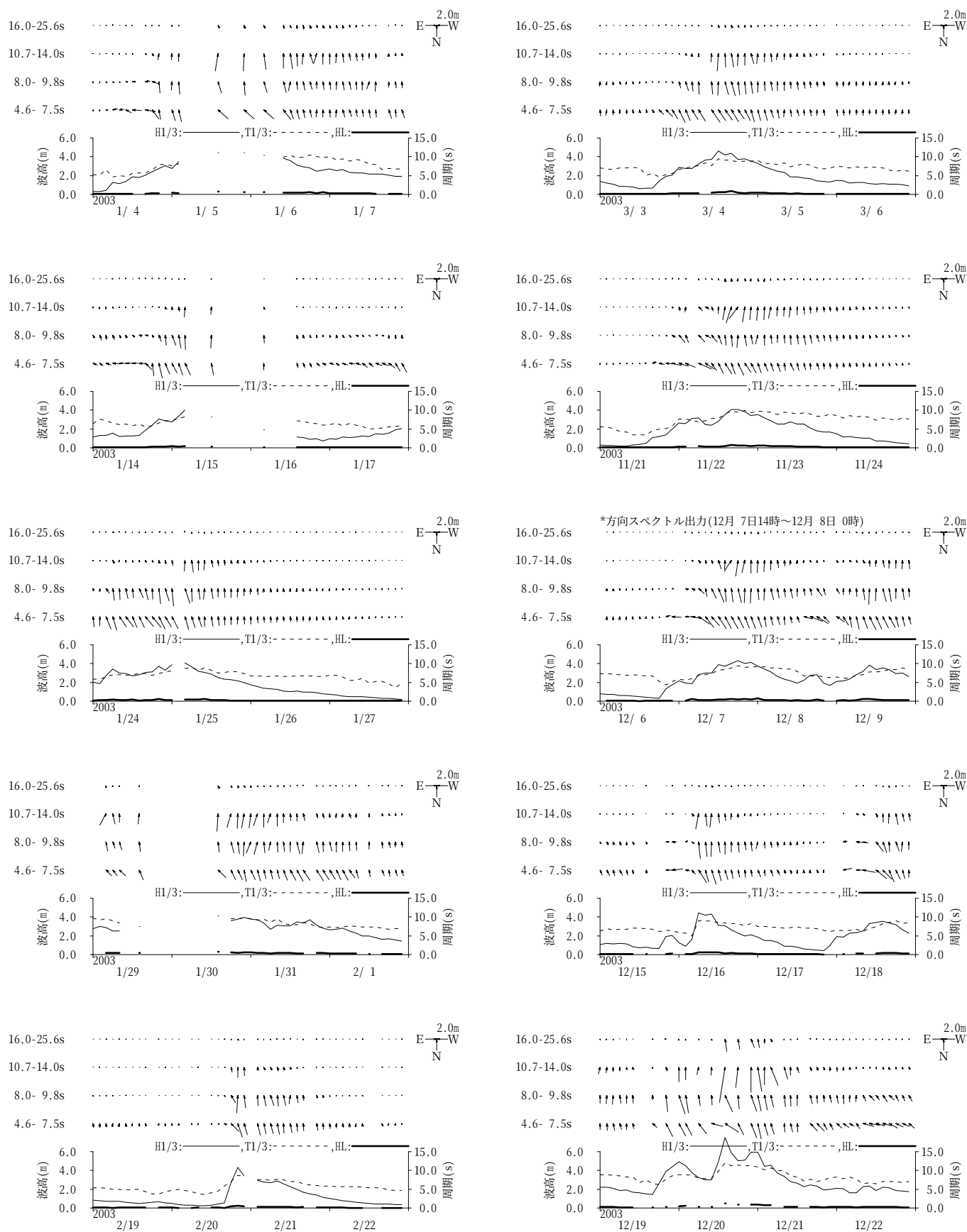
図-11.6 新潟沖 周期帯別波浪特性の経時変化(高波期間中)
