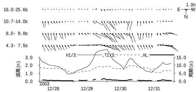
図 - 11.11 金沢 周期帯別波浪特性の経時変化(高波期間中)
