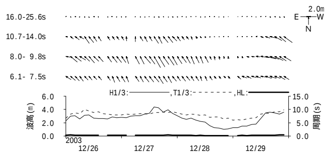
図 - 11.10 輪島 周期帯別波浪特性の経時変化(高波期間中)
