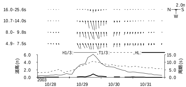
図 - 11.4 秋田 周期帯別波浪特性の経時変化(高波期間中)
