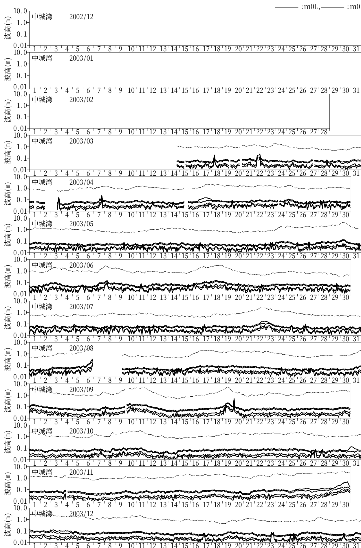
図-10.53 長周期波高の経時変化図（中城湾）
