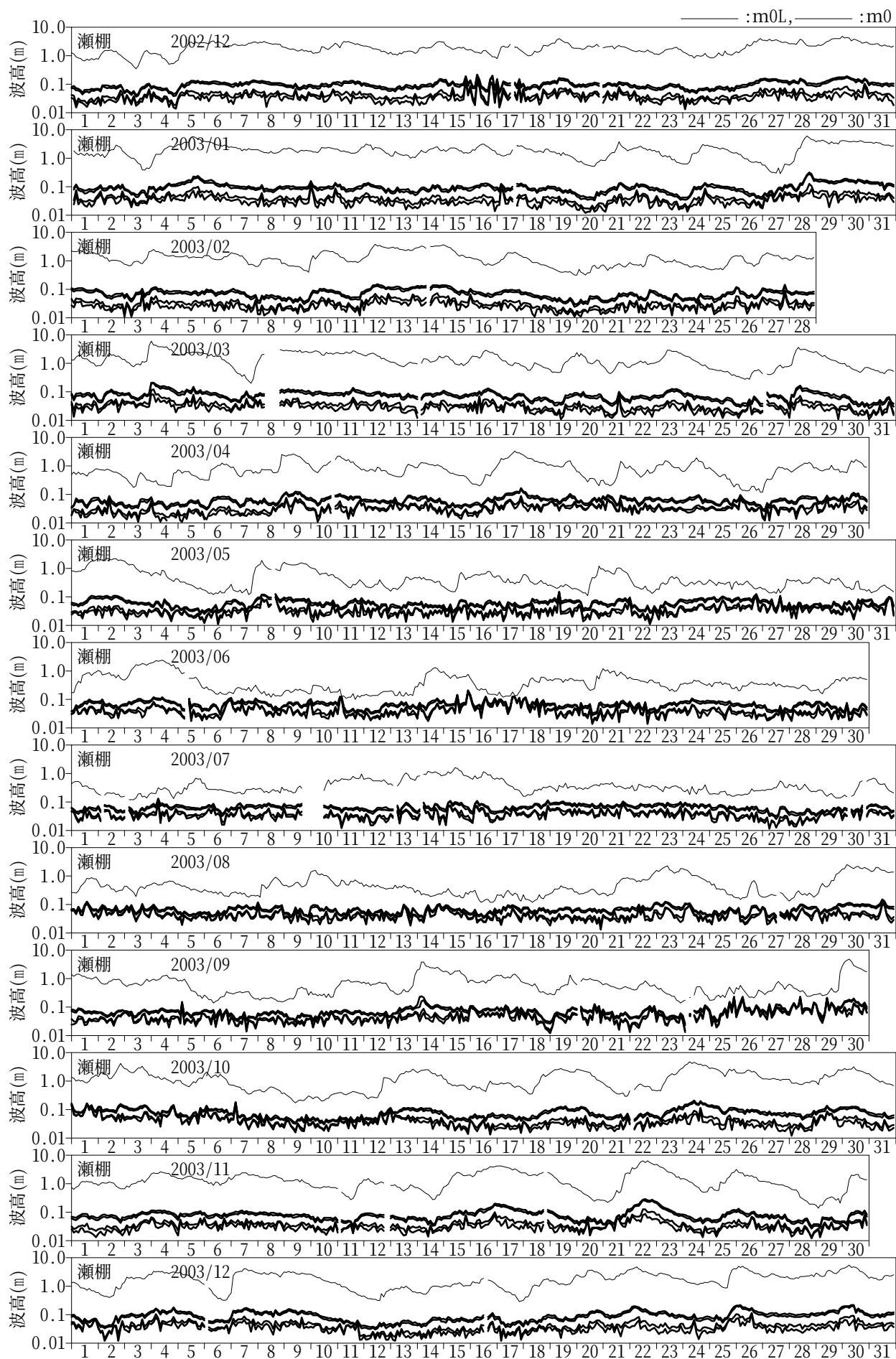
図-10.2 長周期波高の経時変化図（瀬棚）
