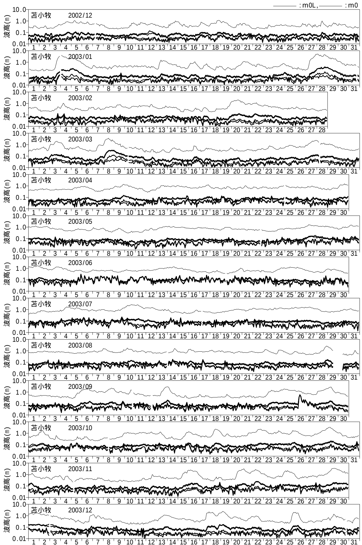
図 - 10.24 長周期波高の経時変化図 (苫小牧)
