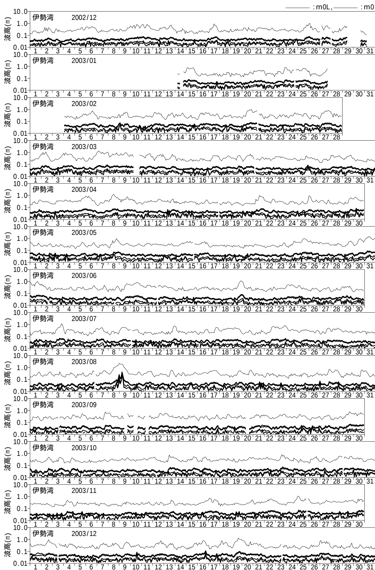
図 - 10.41 長周期波高の経時変化図 (伊勢湾)
