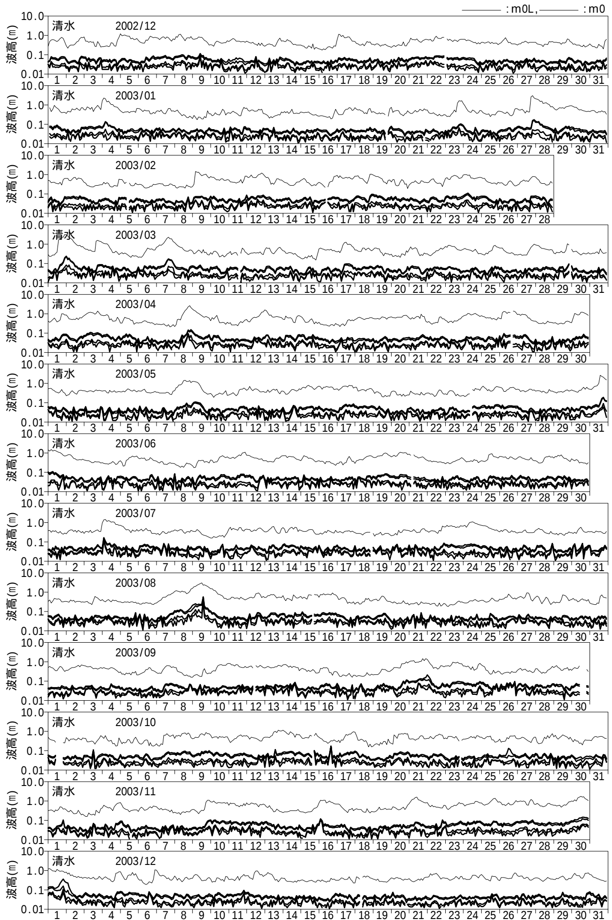
図 - 10.39 長周期波高の経時変化図（清水）
