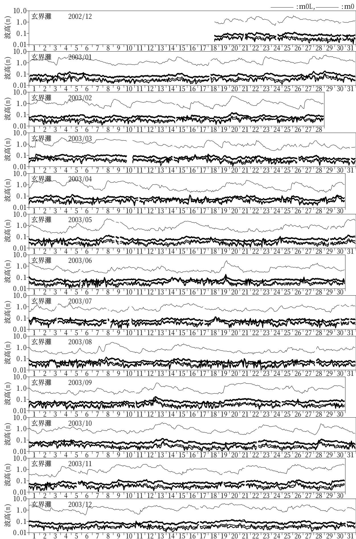
図-10.18 長周期波高の経時変化図（玄界灘）
