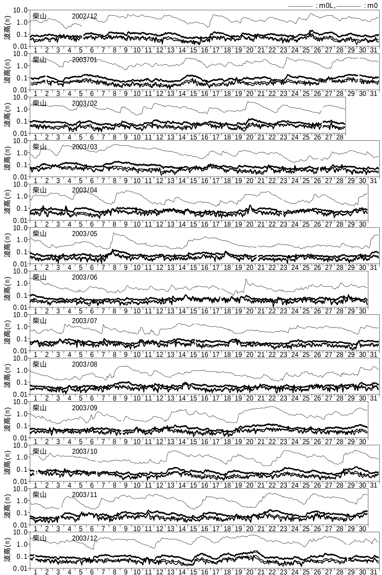
図 - 10.12 長周期波高の経時変化図 (柴山)
